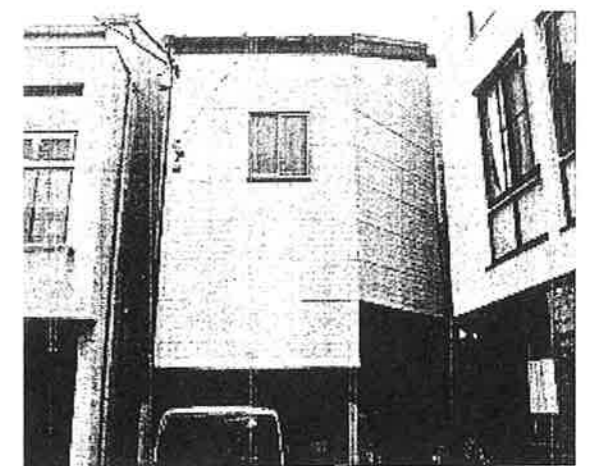
外観 (築年:1995年)
