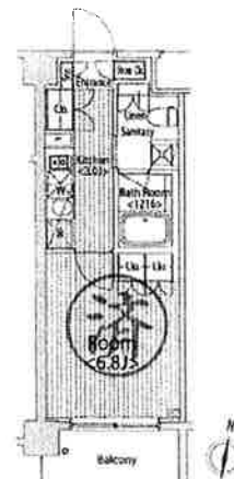
■ E1-type 1K / 25.19㎡[7.61坪]
