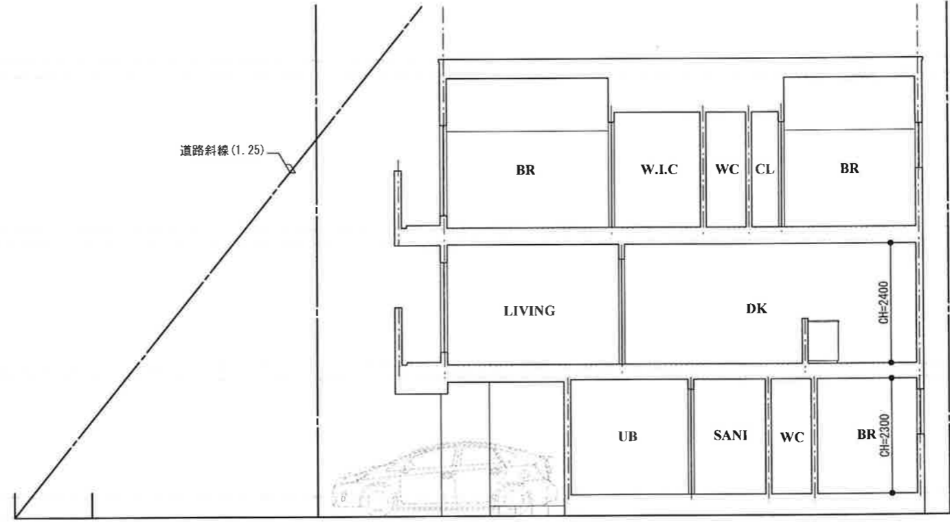
S-N SECTION
